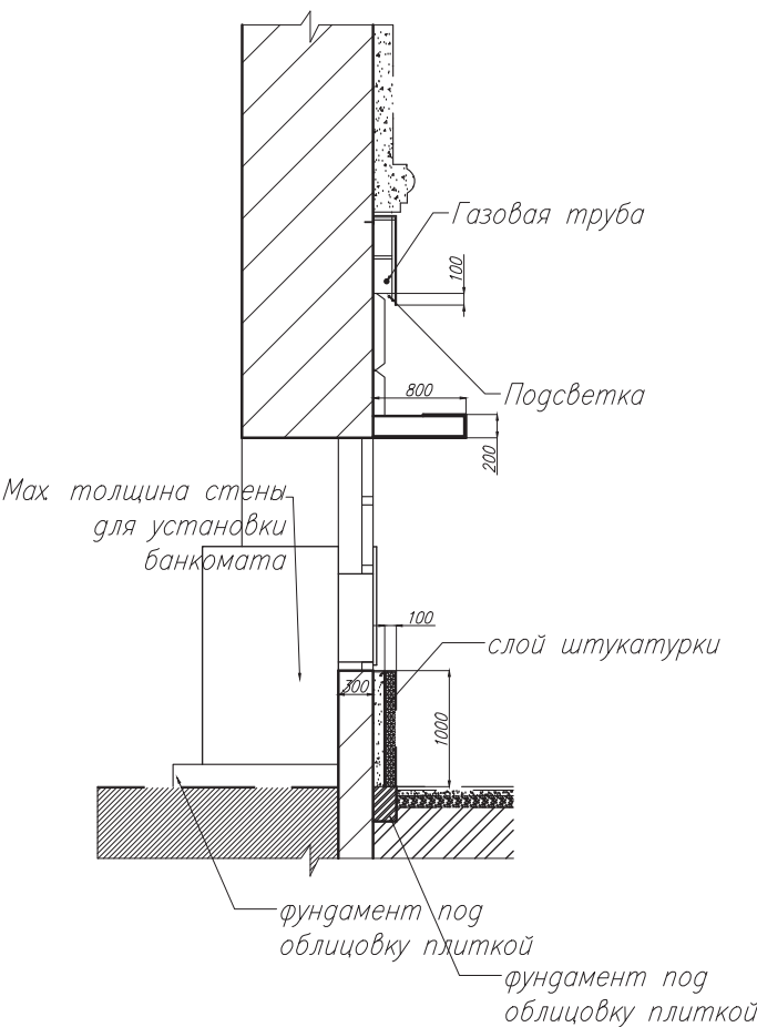
Сечение 4-4
