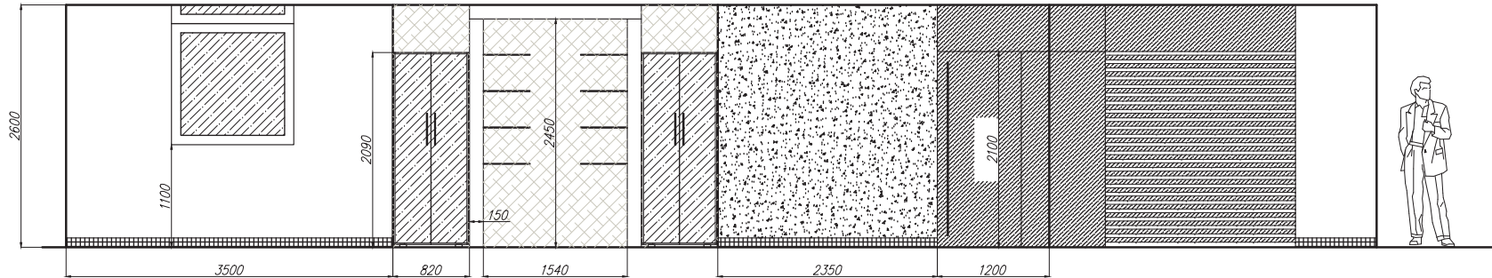
Развертка 2 (Кабинет нач. отдела, вид изнутри)
