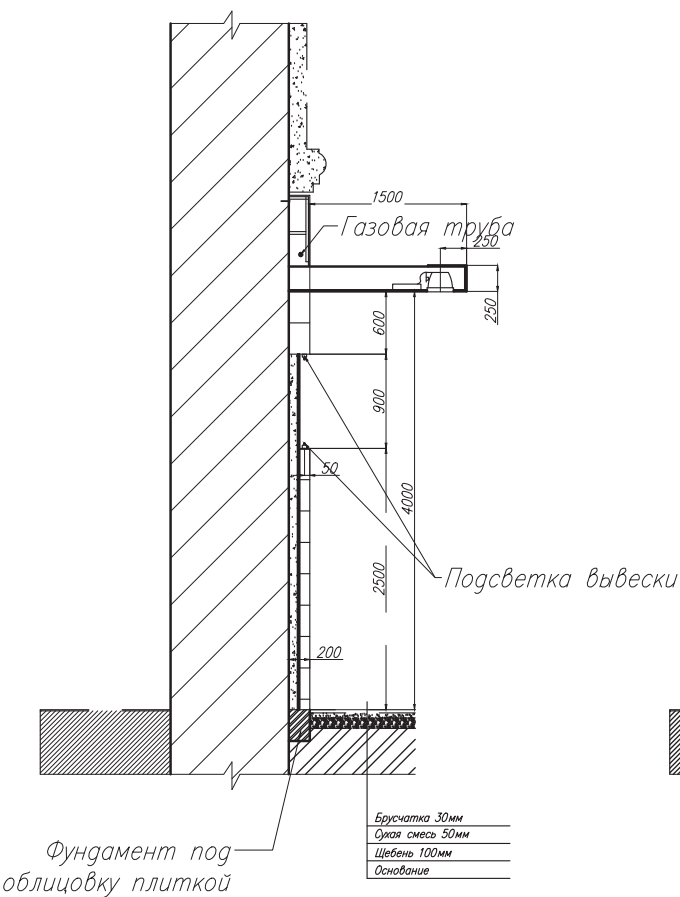
Сечение 1-1
