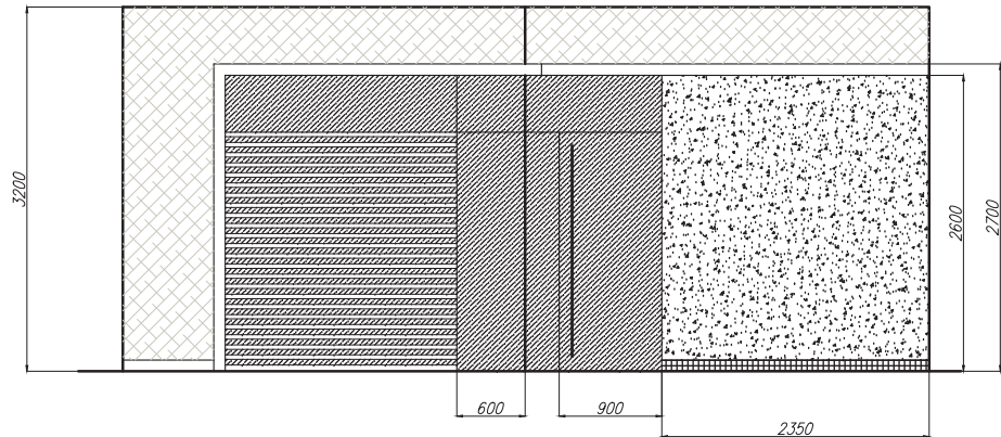
Развертка 3 (Кабинет нач. отдела, вид снаружи)
