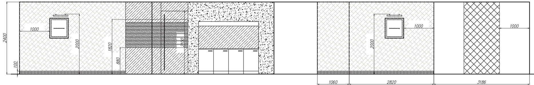
Развертка 1 (Комната переговоров, вид изнутри)
