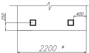
Схема расположения светильников козырька банкомата
