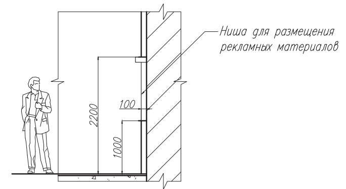
Сечение 3-3
