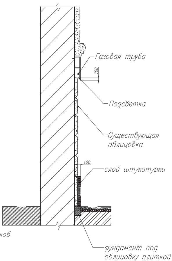
Сечение 3-3
