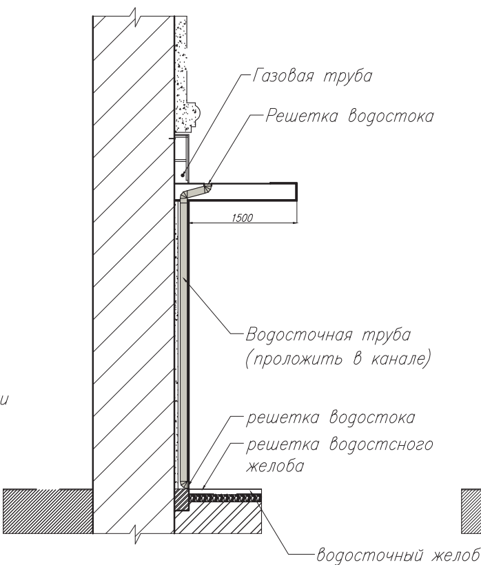
Сечение 2-2
