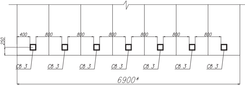
Схема расположения светильников козырька входа
