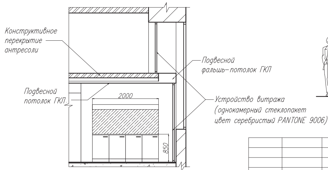
Сечение 4-4
